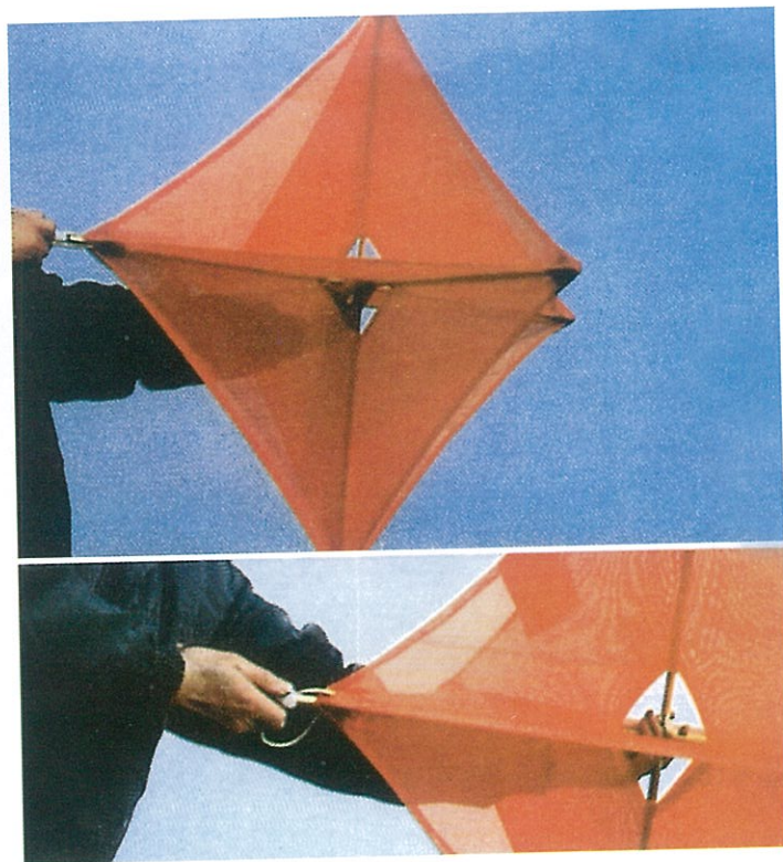
图3 撑开角反射器，使伞弹簧弹出锁定，并旋紧张紧螺栓，以保持反射面的张力。
