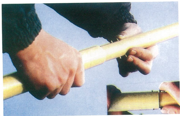
图2 打开包装筒或包装袋，取出角反射器和支柱（由2~3根杆子组成）。连接两杆（救生艇用）或三杆（救生筏用），使连接弹簧销卡牢。
